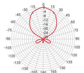
Guadagno (x: frequenza MHz, y: guadagno ISO dBi) e Pattern (@862MHz)
